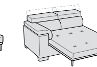
Divano laterale dx/sx letto L 136 P 235 H 76/97
