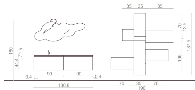
ZERO4_07 / L. 180,8 x P. 51 cm + pensili L. 190 x P. 20,8 cm Scocca e frontali: vetro sabbato blu night con particolari bianco - Piano top in cristallo sabbato bianco sp.1,5 cm con lavabo integrato / Body and fronts: blu night sand-blasted glass with white details - Surface top: sand-blasted white glass th. 1,5 cm with built-in wash-basin.
