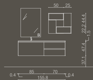
ZERO4_05 / L. 155,8 x P. 51 cm
